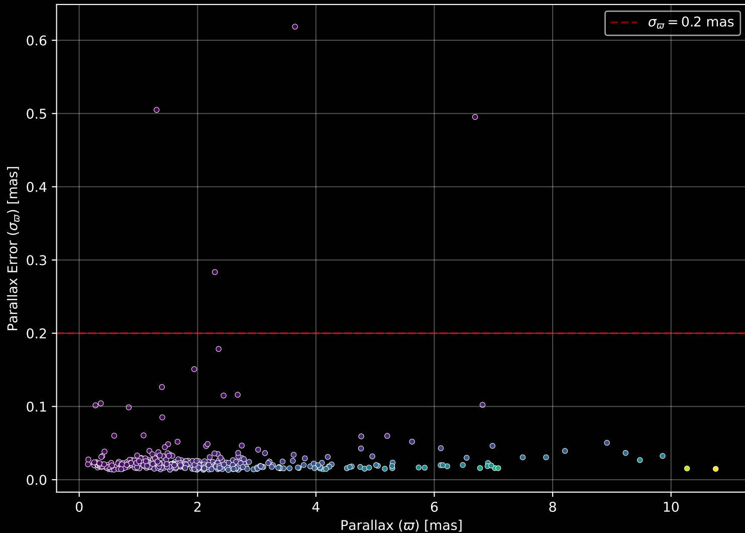
GALAH DR4 Field: [6584] Parallax Quality (n= 409)
