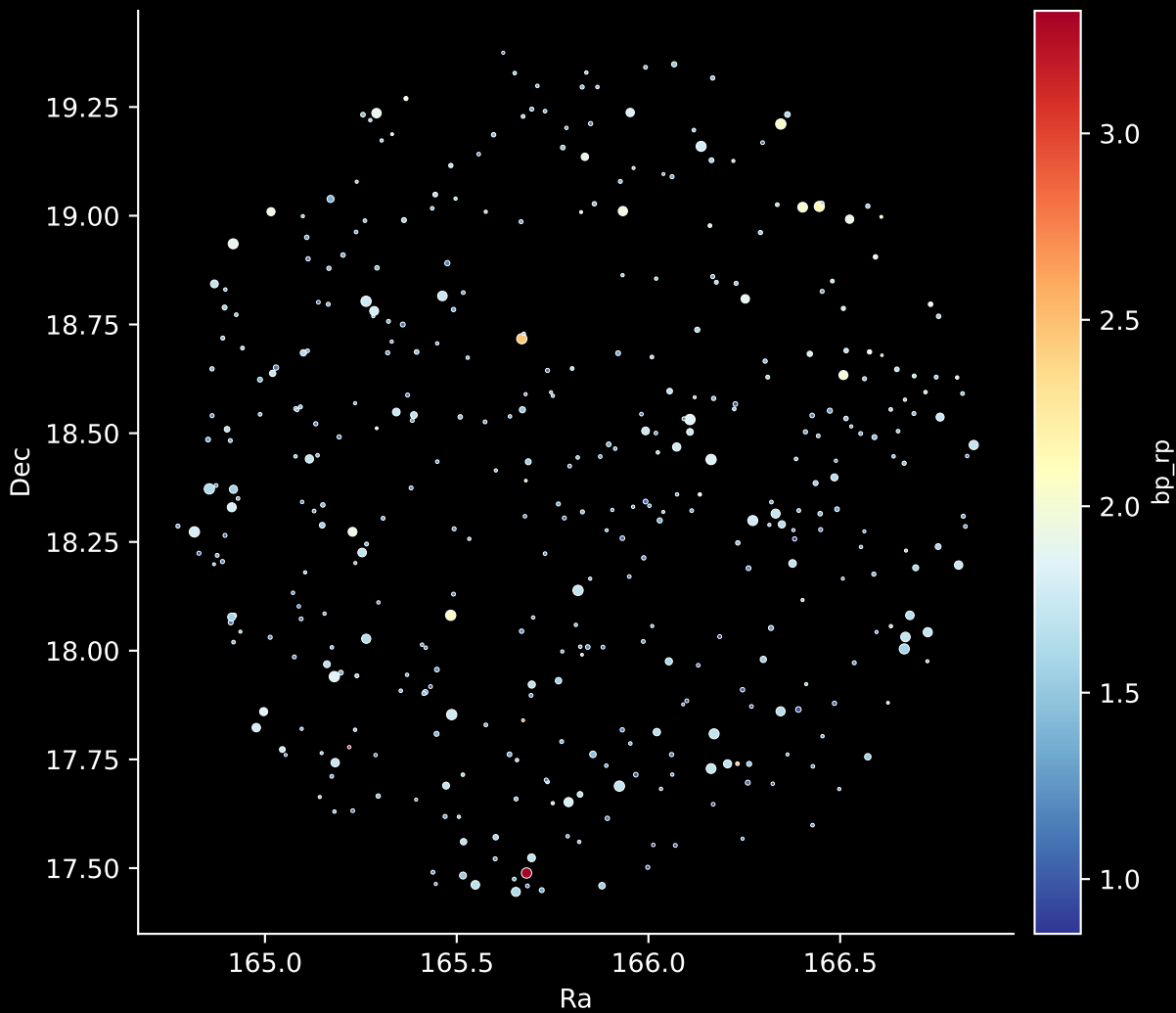
GALAH DR4 Field: [6584] Stars: 409
